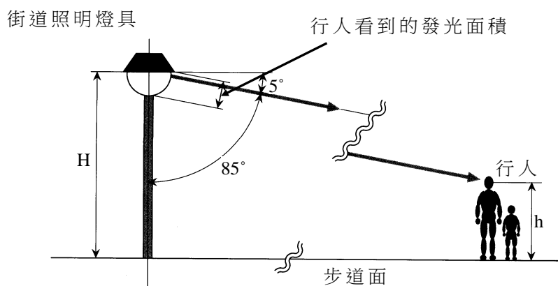
圖 2 街道照明燈具與行人間之位置示意圖
